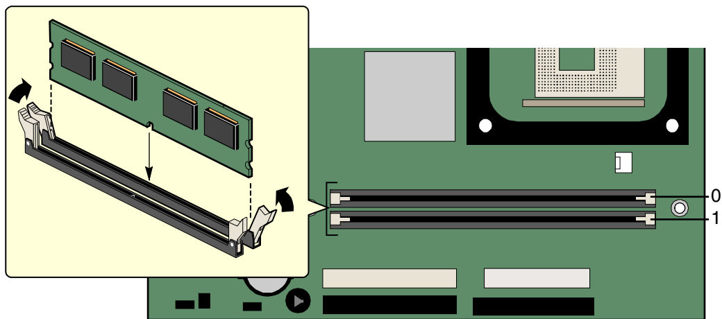
图 7. 安装 DIMM
