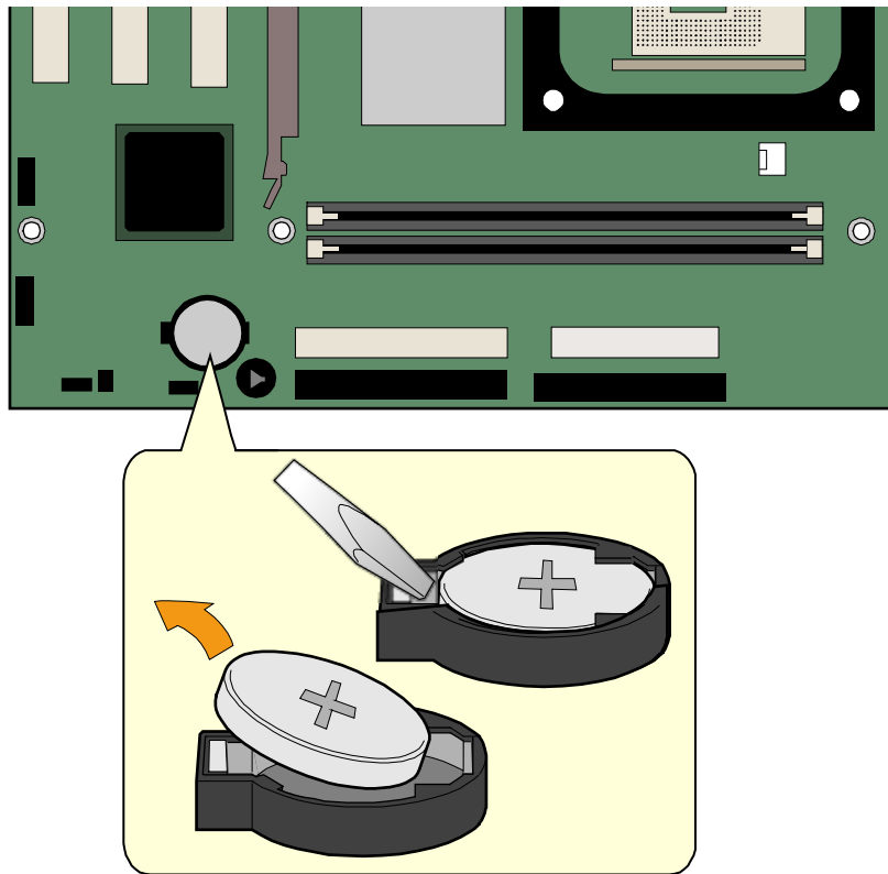
图 14. 从桌面主板上拆卸电池
