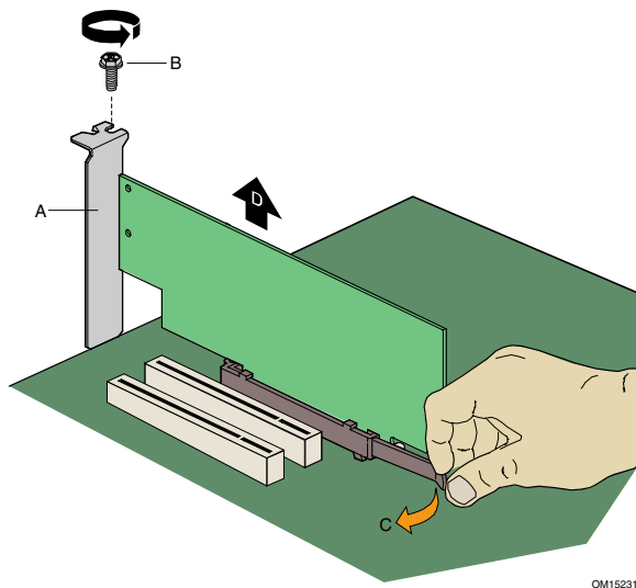
图 6. 拆卸 AGP 卡
