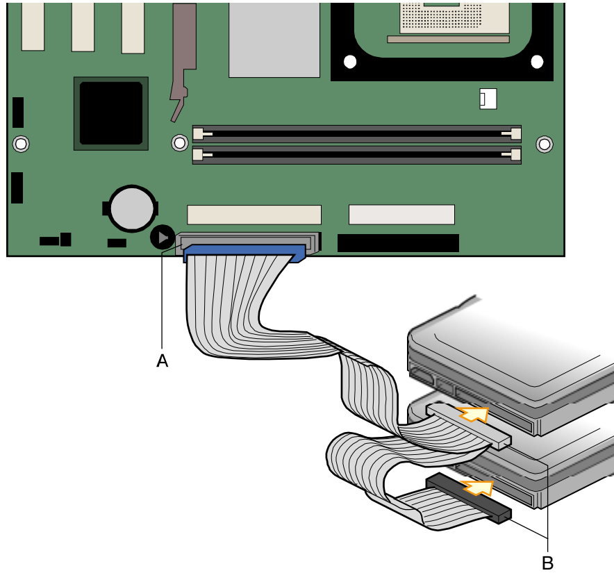
图 8. 连接 IDE 电缆
