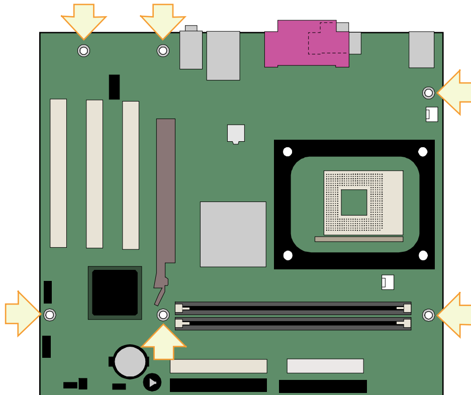
图 3. 桌面主板安装螺丝孔位
