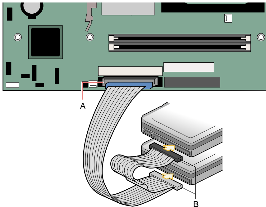
图 9. 连接 IDE 电缆
