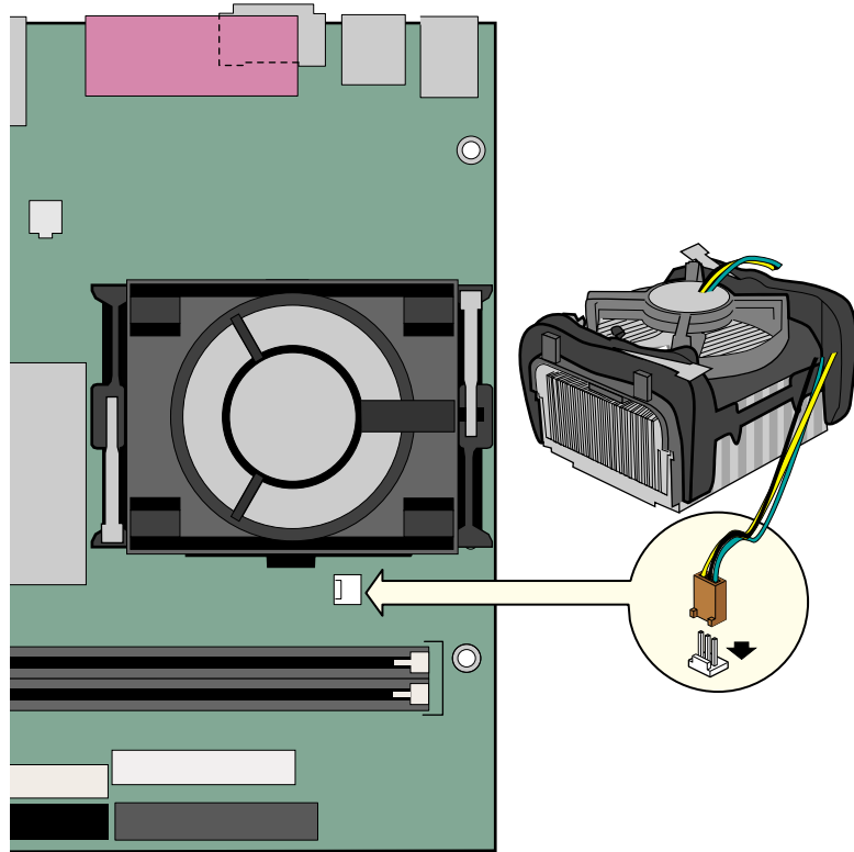
图 6. 将处理器风扇散热器电缆连接到处理器风扇连接器上
