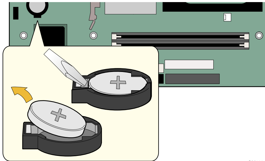
图 15. 拆卸电池
