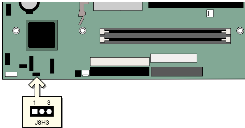
图 14. BIOS 配置跳线块的位置
