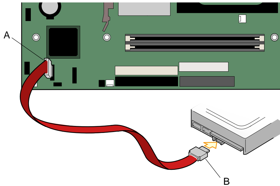
图 10. 连接串行 ATA 电缆
