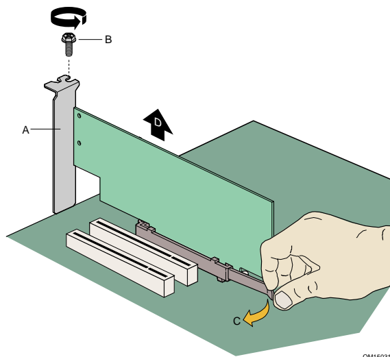
图 8. 拆卸 AGP 卡
