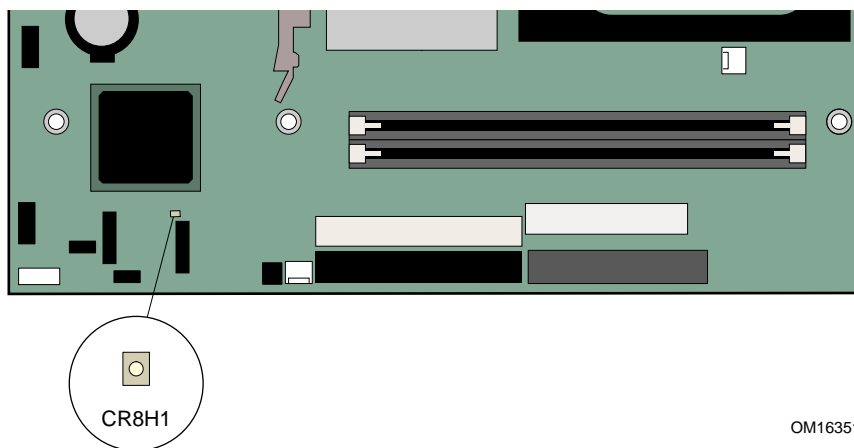
图 2. 备用电源指示灯位置
