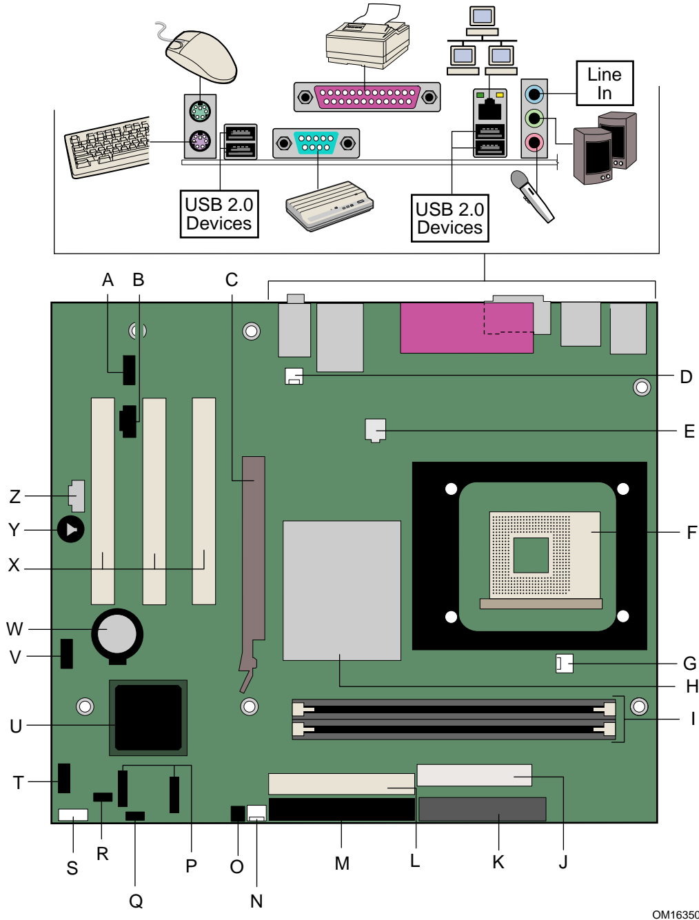
图 1. 桌面主板组件
