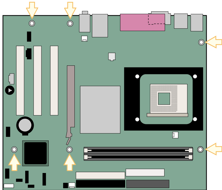
图 4. 桌面主板安装螺丝孔位置
