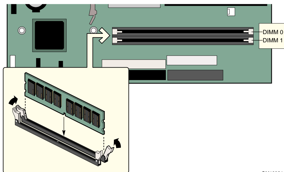
图 7. 安装内存模块
