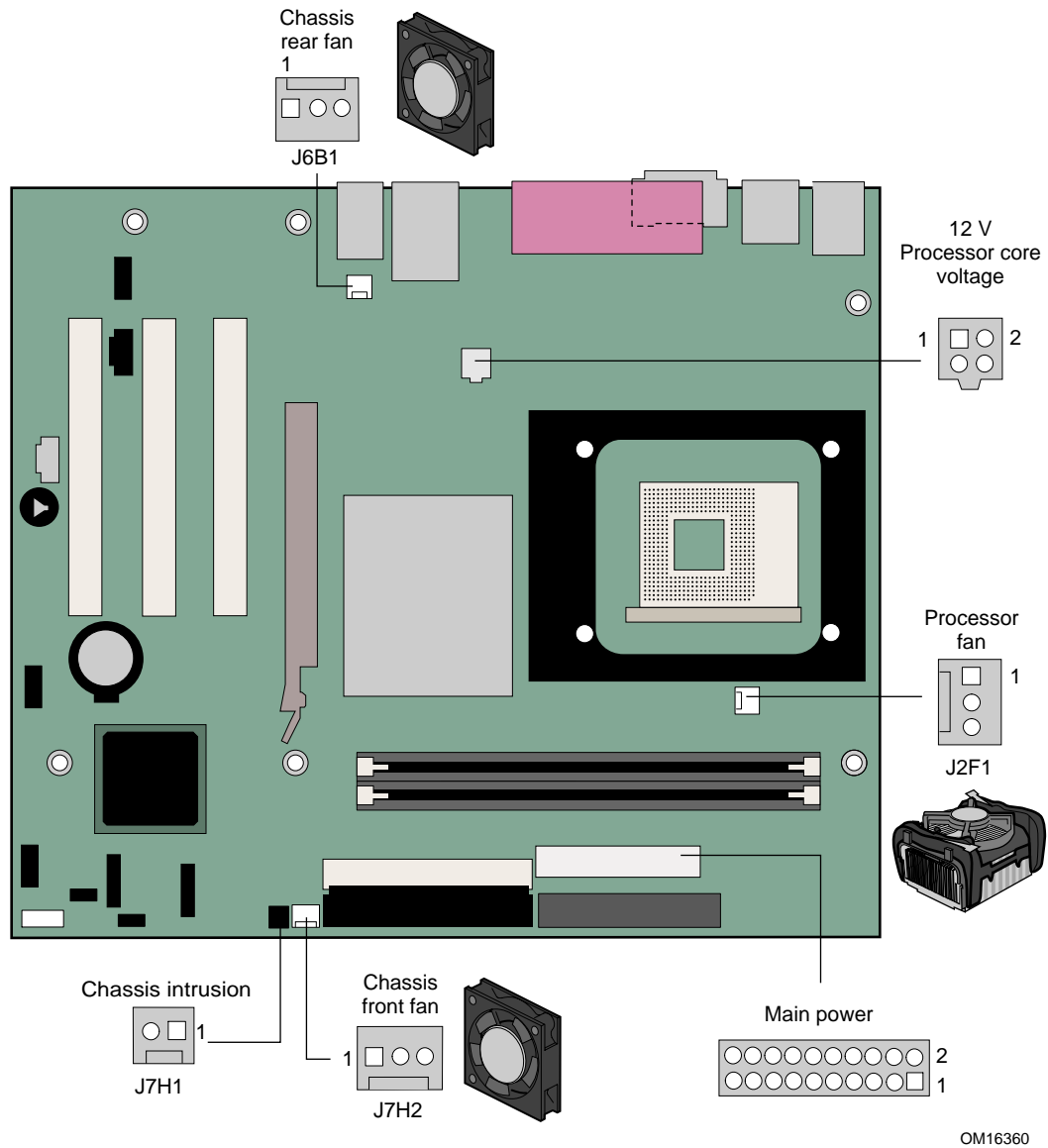
图 13. 硬件控制接头连接器和电源连接器的位置
