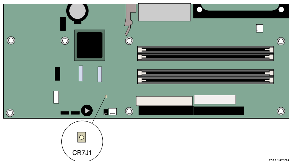
图 2. 备用电源指示灯的位置
