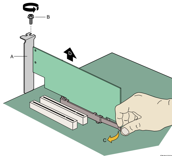
图 10. 拆卸 AGP 卡
