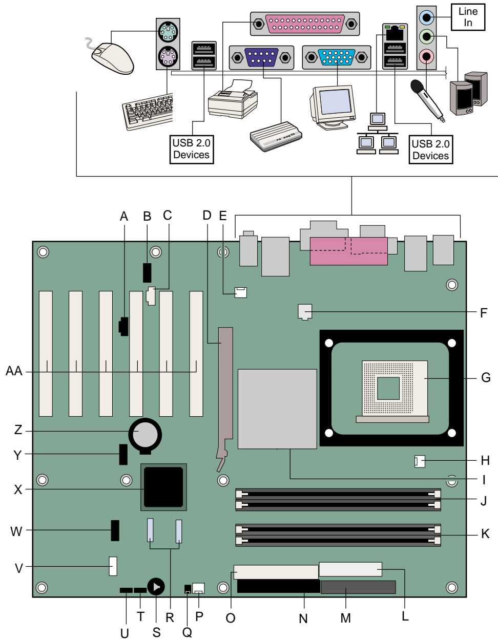
图 1. 桌面主板 D865GBF 组件
