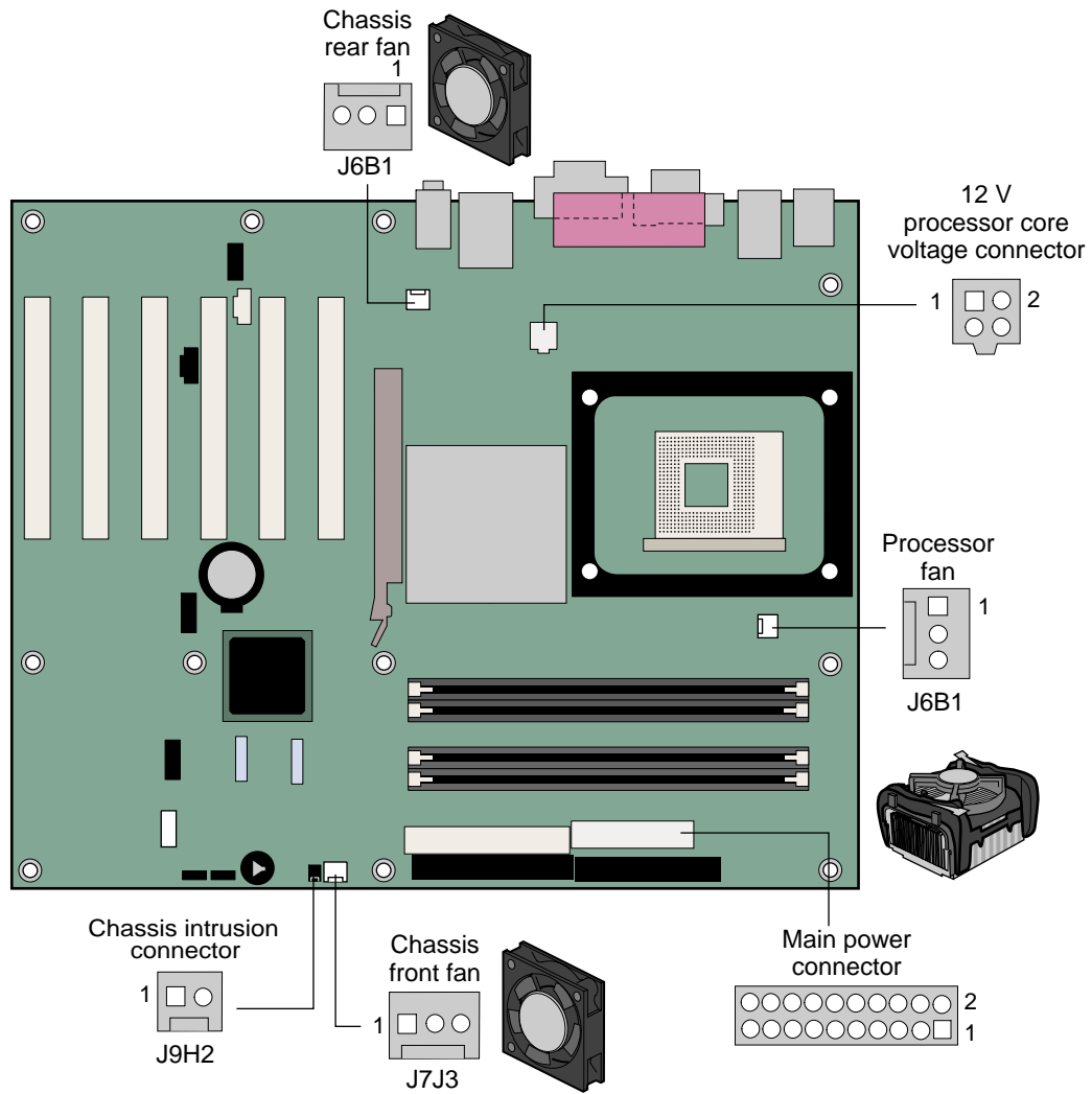
图 15. 硬件控制接头连接器和电源连接器的位置
