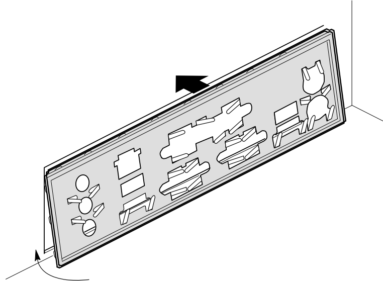
图 3. 安装 I/O 防护板
