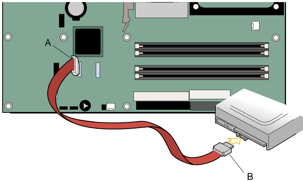
图 12. 连接串行 ATA 电缆
