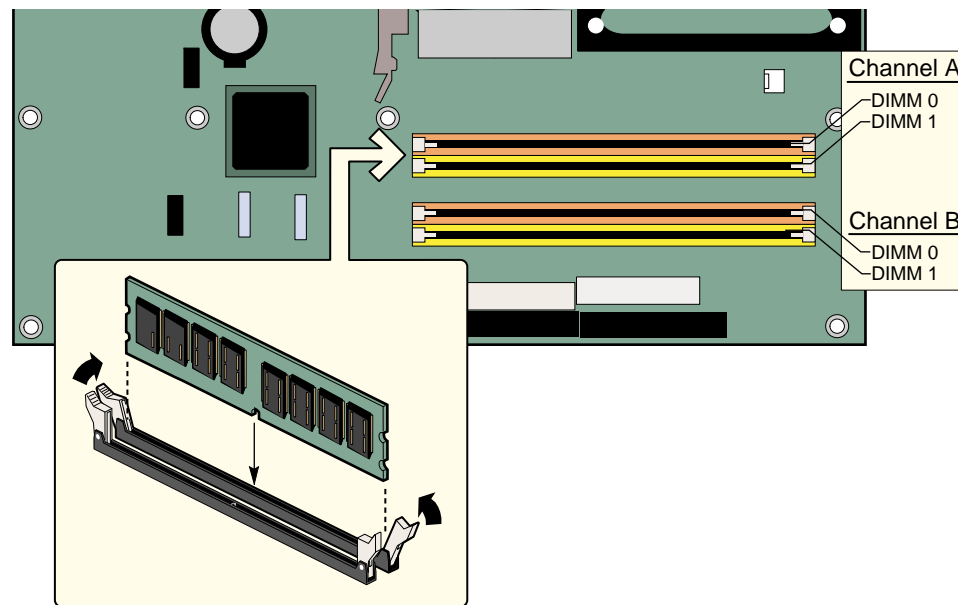
图 7. 安装内存模块
