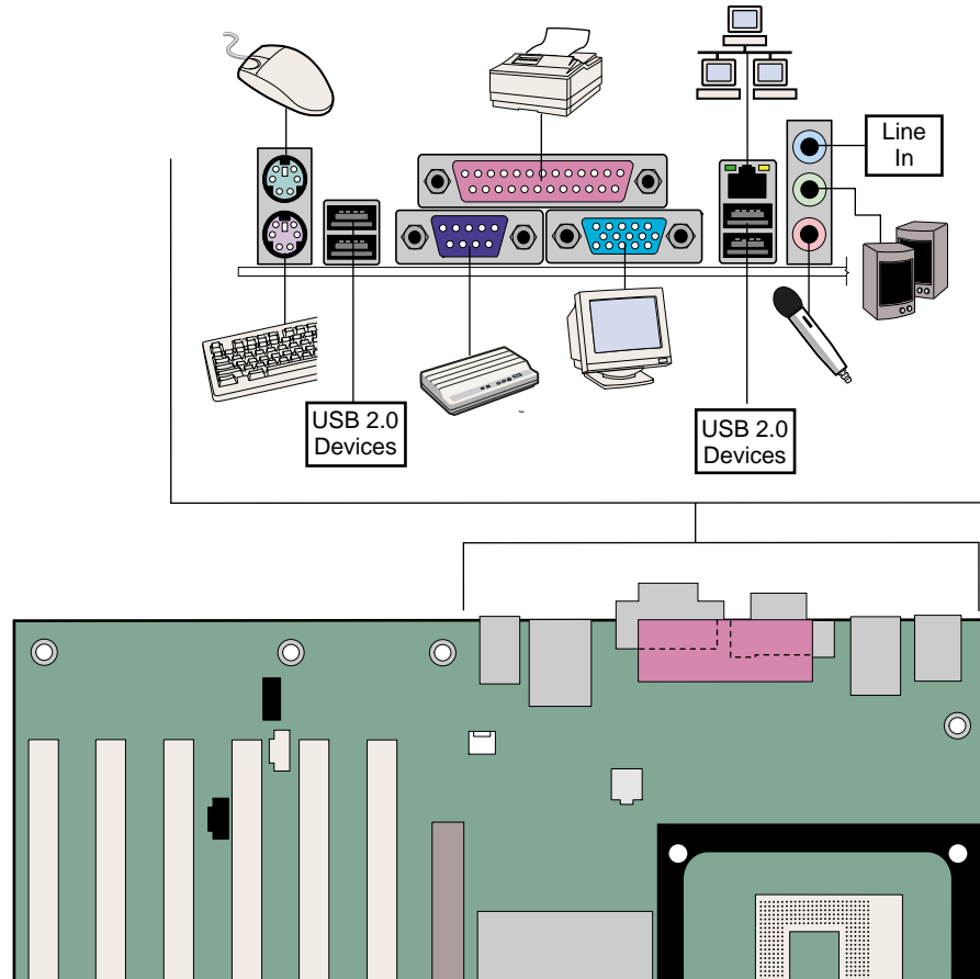
图 18. 背面板连接器
