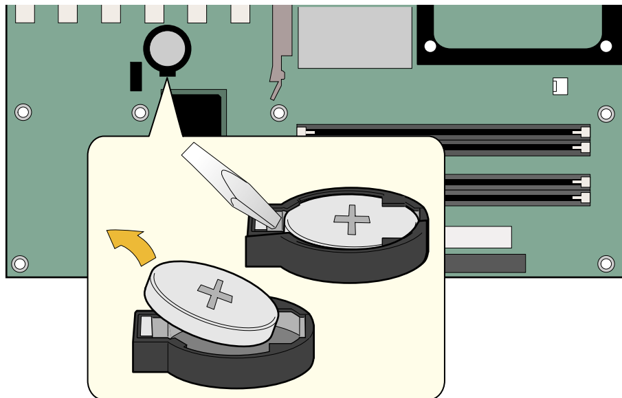
图 17. 拆卸电池
