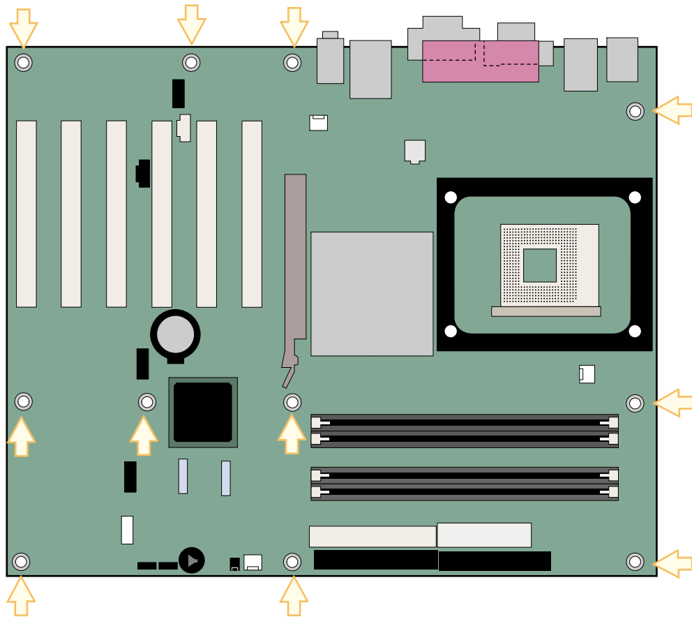
图 4. 桌面 motherboard 安装螺丝孔位置
