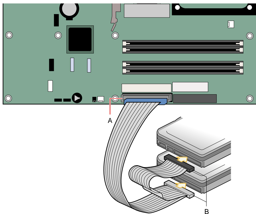
图 11. 连接 IDE 电缆
