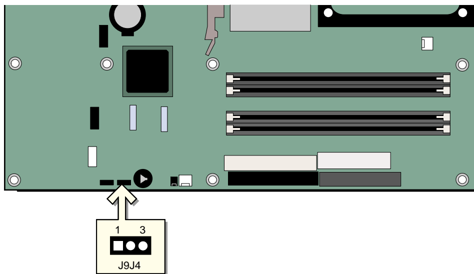
图 16. BIOS 配置跳线块的位置
