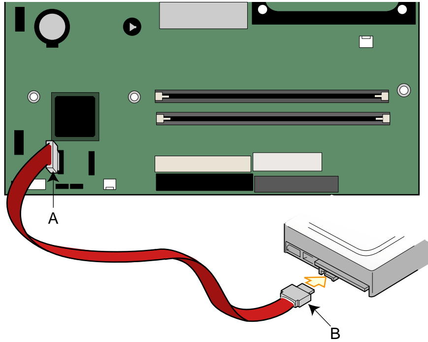
图 8. 连接串行 ATA 电缆
