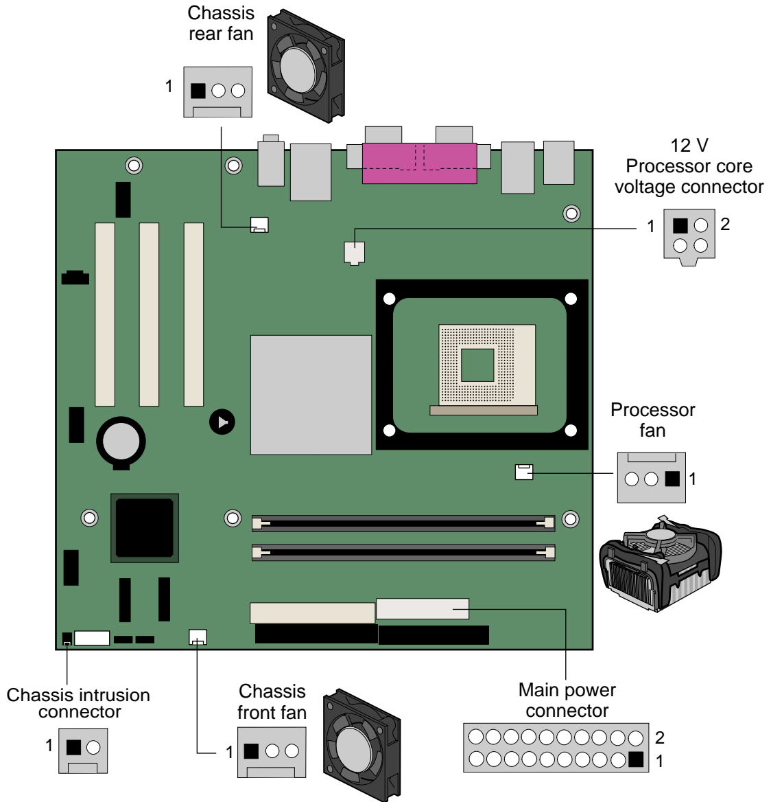
图 10. 硬件控制接头连接器和电源系统连接器的位置
