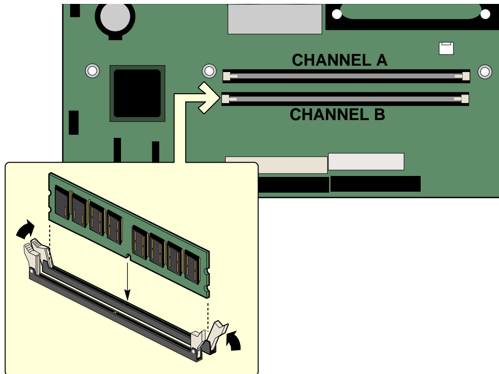
图 6. 安装内存模块
