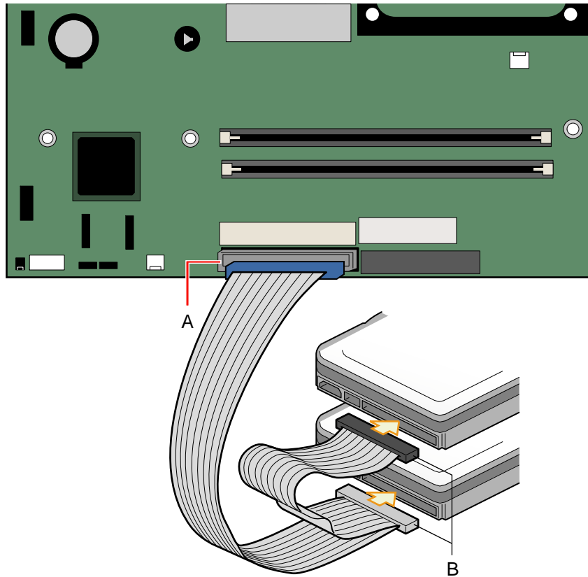
图 7. 连接 IDE 电缆
