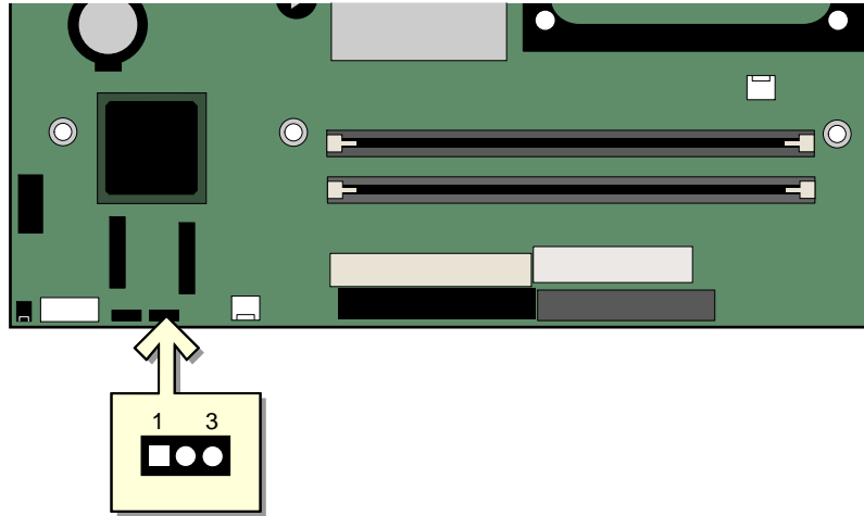
图 12. BIOS 配置跳线块的位置
