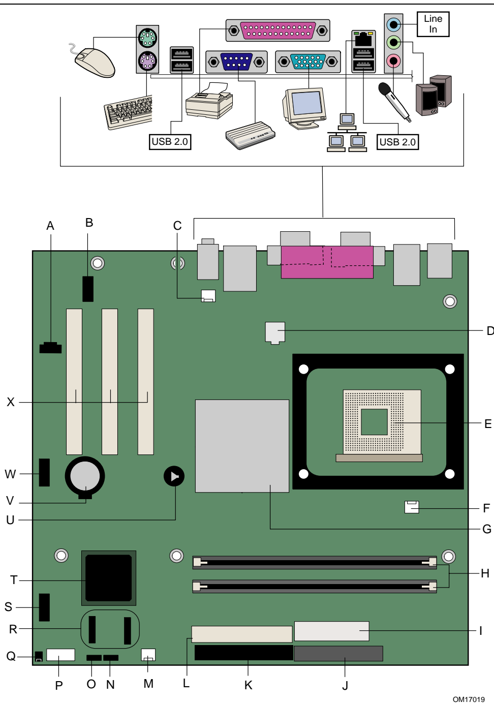
图 1. 桌面主板 D865GVHZ 组件
