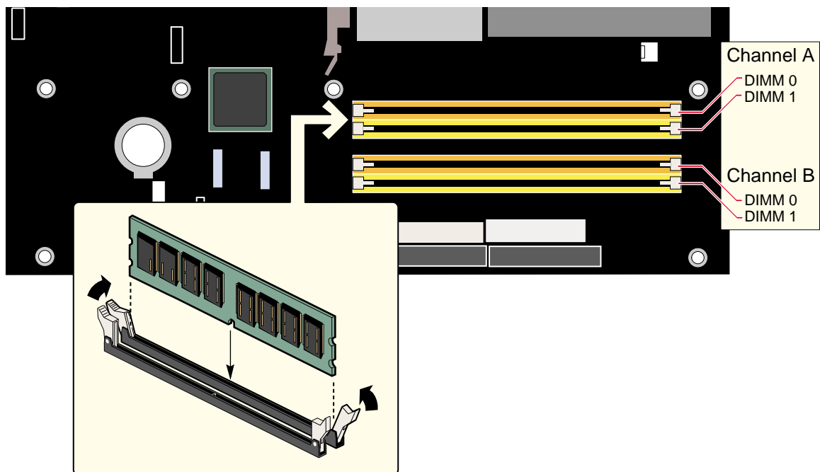
图 9. 安装内存模块
