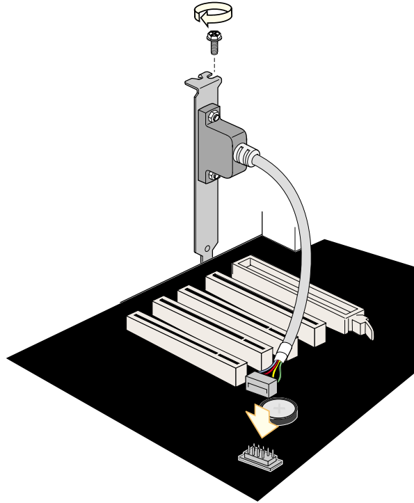
图 14. 连接背面板 USB 2.0 适配器
