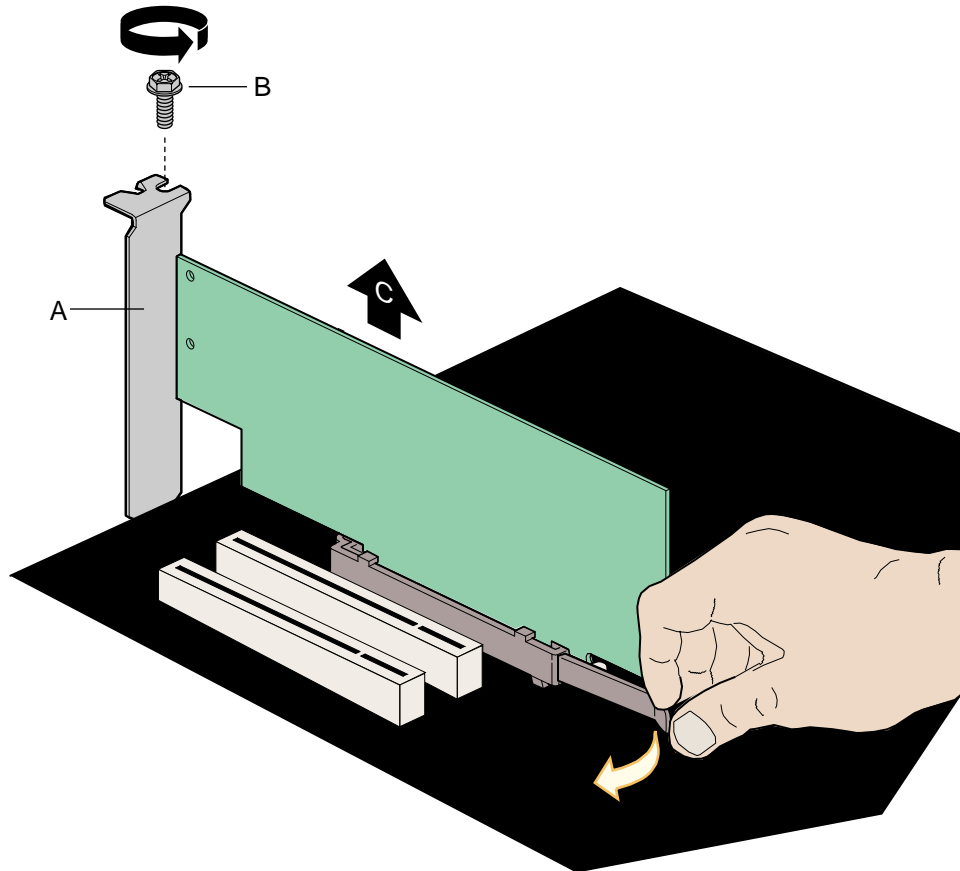
图 10. 拆卸 AGP 卡
