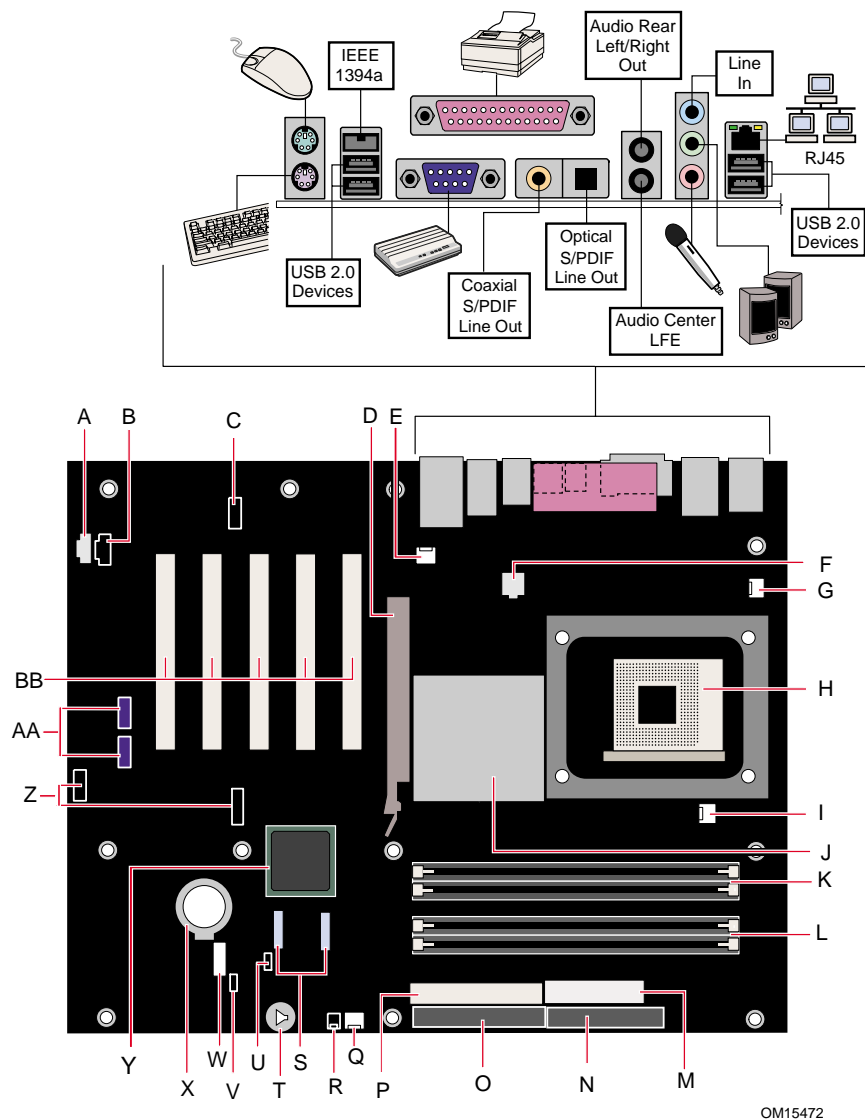
图 1. 桌面主板 D865PERL 组件
