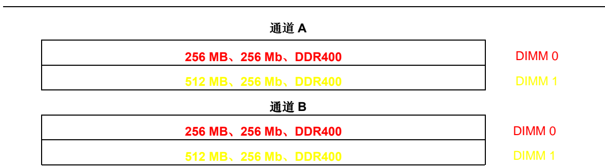
图 8. 双通道配置示例 2
