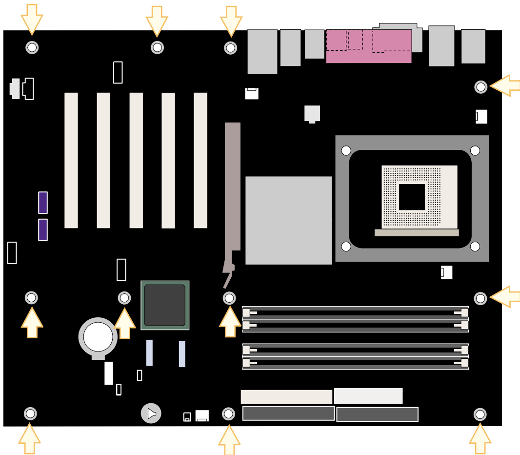
图 4. 桌面主板安装孔位置
