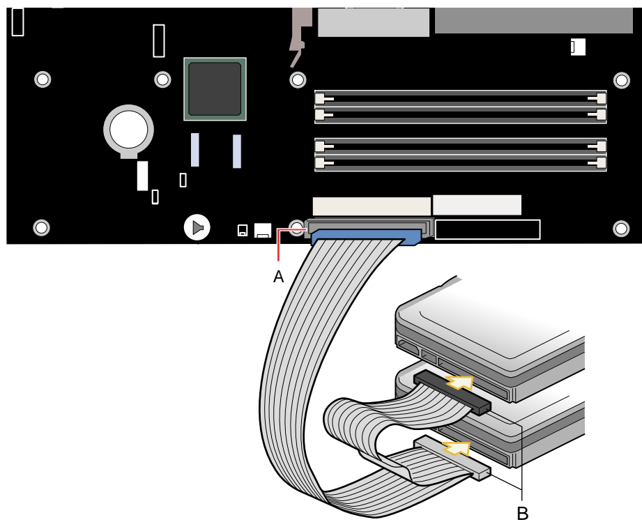
图 11. 连接 IDE 电缆
