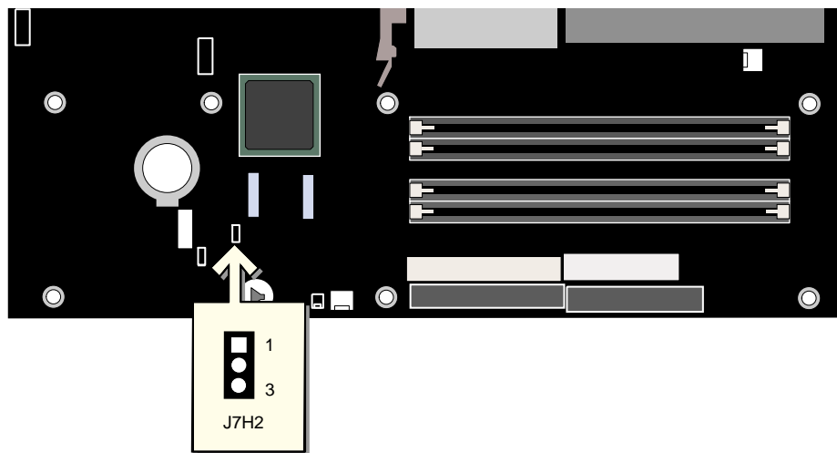
图 18. BIOS 配置跳线块的位置
