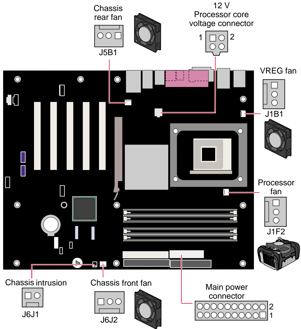
图 17. 硬件控制和电源连接器的位置
