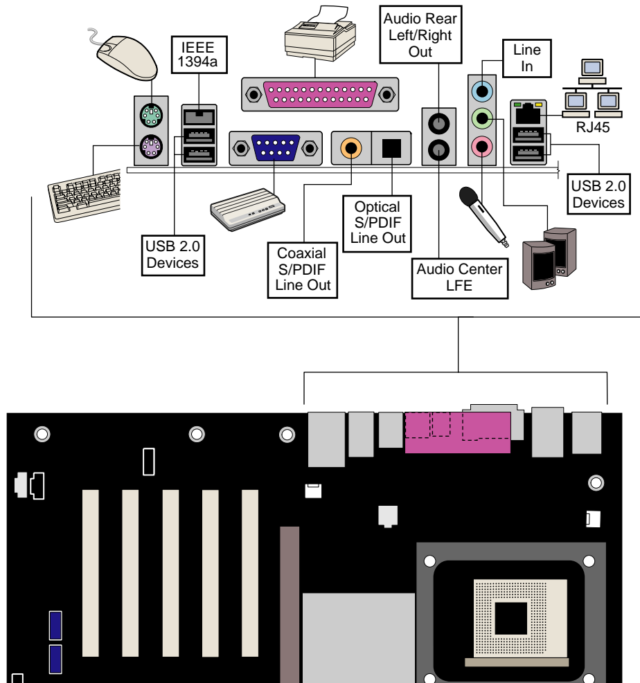
图 20. 背面板连接器
