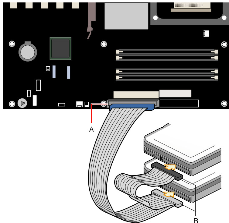
图 11. 连接 IDE 电缆
