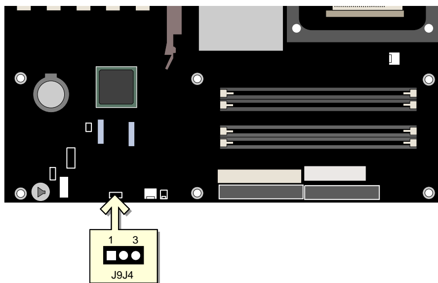
图 15. BIOS 配置跳线块的位置
