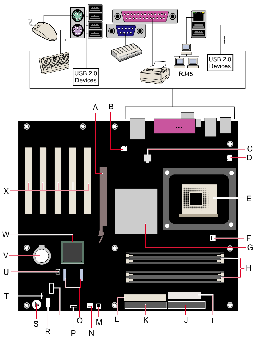
图 1. 桌面主板组件
