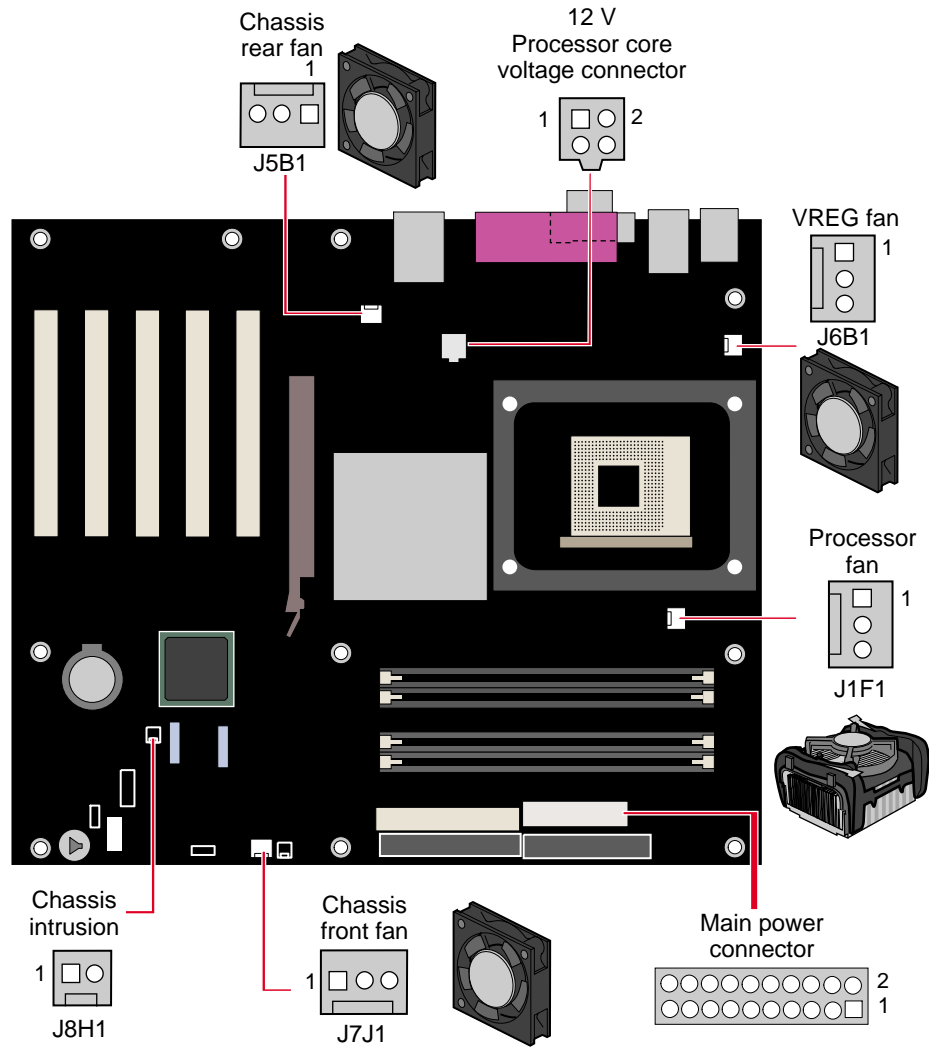
图 14. 硬件控制接头连接器和电源连接器的位置
