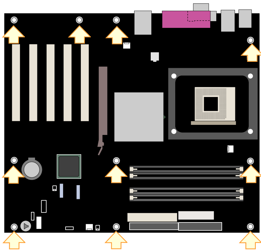
图 4. 桌面主板固定螺丝的安装孔位置
