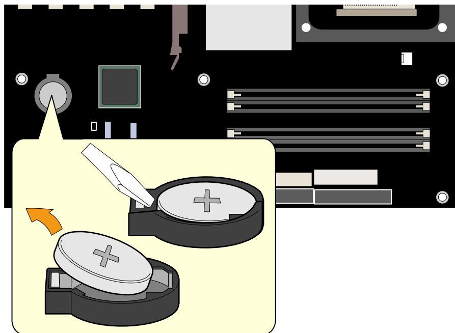
图 16. 更换电池
