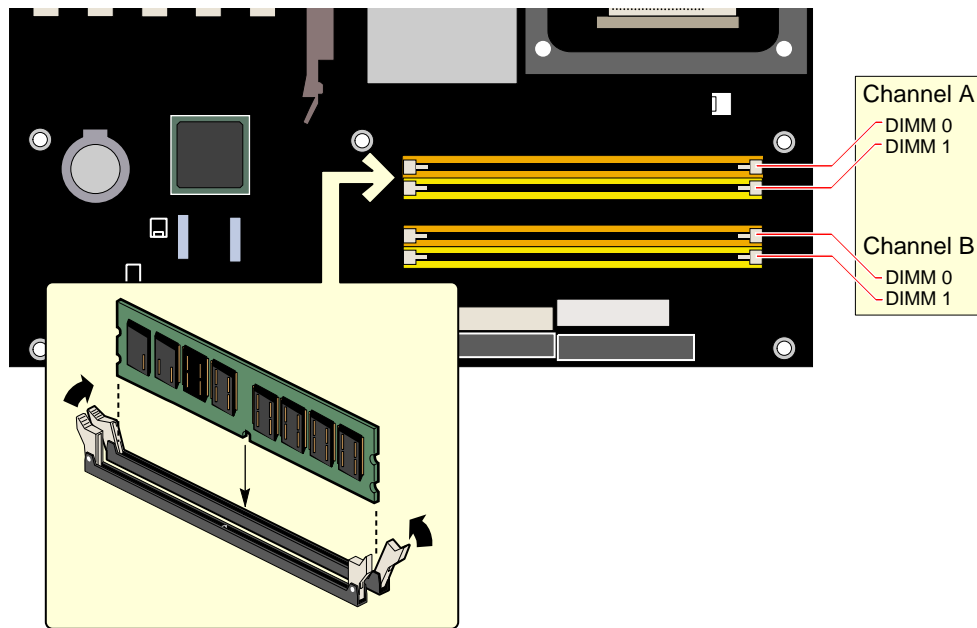
图 7. 安装 DIMM
