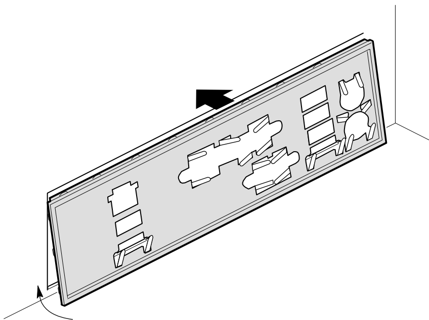
图 3. I/O 防护板
