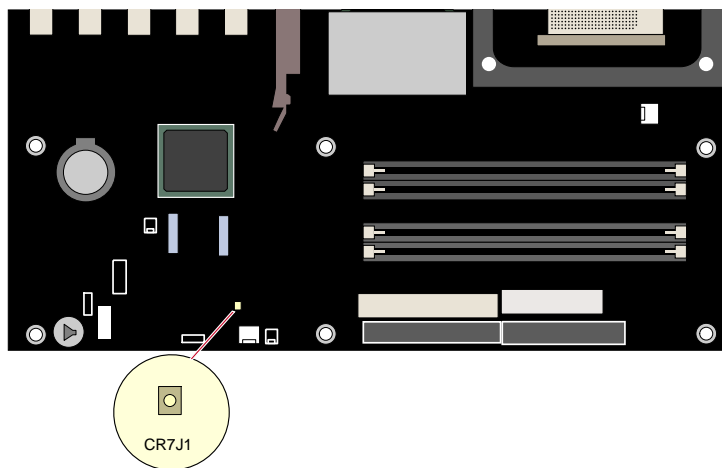
图 2. 备用电源指示灯的位置
