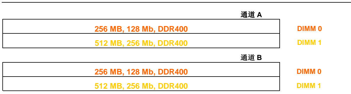
图 9. 使用四条 DIMM 的双通道配置示例
