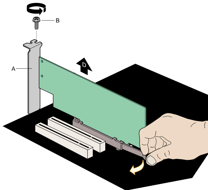
图 10. 拆卸 AGP 卡
